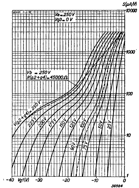
Fig. 13 Steilheid als functie van de negatieve roosterspanning van het heptodegedeelte bij V_a = 250 V en V_{g_3} = 0 V, met de schermroosterspanning als parameter.
