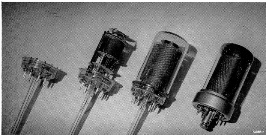
Fig. 1 Vier stadia uit de montage van de triode-heptode steutelbuis ECH 21
