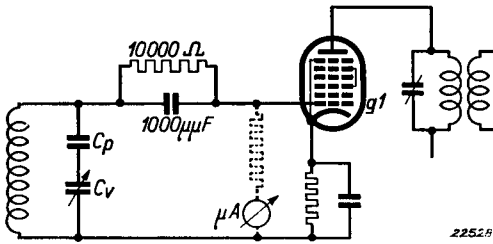
Abb. 11 Schaltung bei Verwendung eines kleineren Ableitwiderstandes (10.000 Ω). Es ist auch angegeben, wie man die Oszillatoramplitude durch Gitterstrom messen kann.
