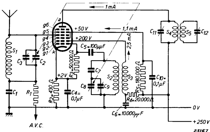
Abb. 10 Prinzipschaltung der Oktode EK 2.
